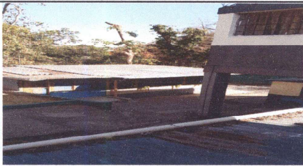
Foto 9: Mantenimiento de estructura de metal donde se colocará nueva lámina troquelada de aluzinc calibre 26, lijada con fondo gris y aplicación de pintura roja en aula de 3ro. Primaria Sección A
