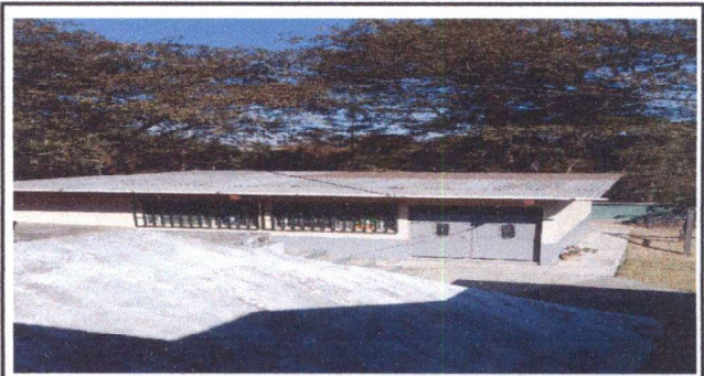
Foto 2: Sustitución de lámina de zinc acanalada que se encuentra con mucho óxido por lámina de aluzinc troquelada calibre 26 en grado de 4to. Primaria Sección A
