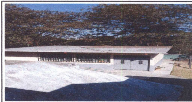
Foto 10: Sustitución de canal de PVC a canal rectangular de 20x15x240 de alto caudal aluzinc calibre 26 con pendientes en el canal en aula de 4to. Primaria Sección A
