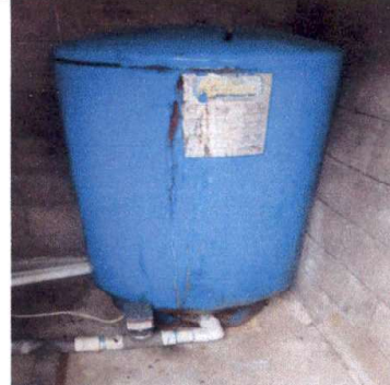
Foto 2: Tanque de 85 galones con perforaciones que ha sido reparado continuamente y está a punto de colapsar. Es un accesorio de la bomba de agua.
