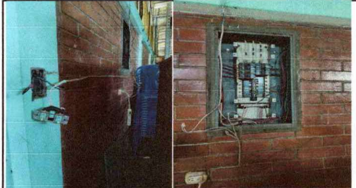
Foto2: REPARACIÓN DE SISTEMA ELÉCTRICO EN TALLERES DE COCINA
