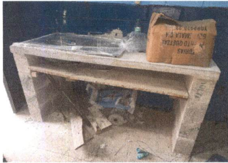
Foto1: RENGLÓN INSTALACIÓN LAVATRASTOS EN COCINA
