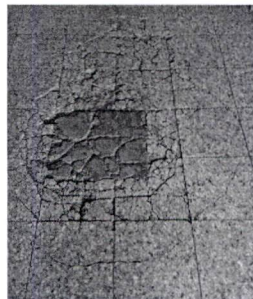
Foto1: Sustitución de piso de granito de 25.6 Mts.2
