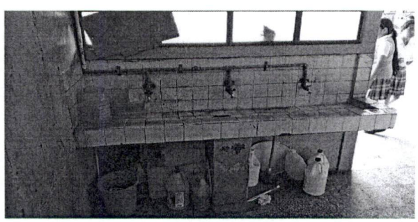
FOTO 9: Reparación de lavamanos multiple e instalación de grifería nueva
