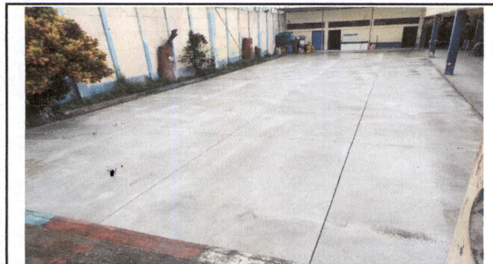
Foto 1: Reparación de planchas de concreto en patio central (Losa de patio)
