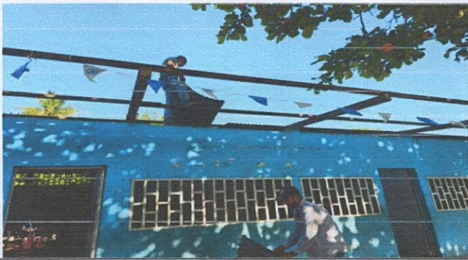
Foto1: SUSTITUCION POR LAMINA, POR LAMINA TROQUELADA ALUZING 26
