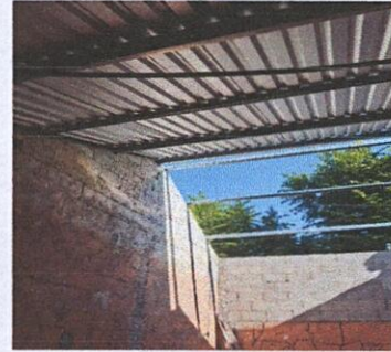
FOTO 2: ESTRUCTURA DE TECHO (sustitución de estructura de soporte de metal, por metal)
