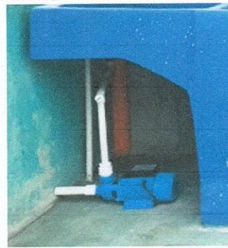
Foto 11: REPARACION Y MANTENIMIENTO DE CISTERNAS Y DEPOSITO DE AGUA. 18.3 Sustitución de bomba de agua
