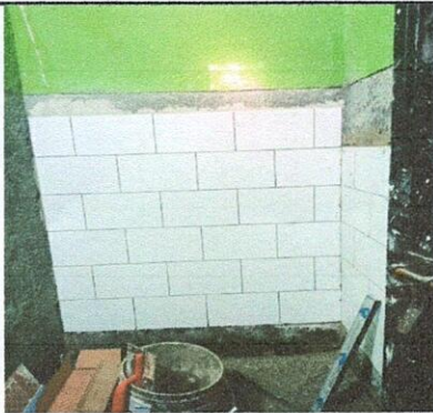
Foto 08: SUSTITUCION DE AZULEJO. 13.1 Sustitución de azulejo
