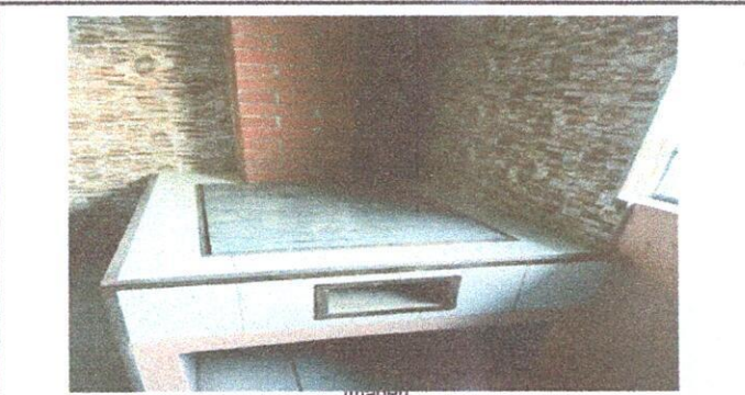
Foto13: 20. REPARACIÓN DE COCINA. 20.3 Sustitución de plancha de metal de 3 hornillas, 20.7 Instalación de azulejo en estufa rural.
