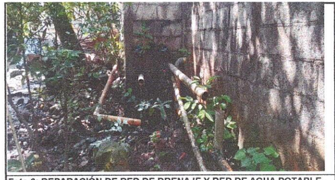
Foto 6: REPARACIÓN DE RED DE DRENAJE Y RED DE AGUA POTABLE. 14.3 Sustitución de tubería PVC línea principal de aguas negras. 14.8 Sustitución de caja de registro.
