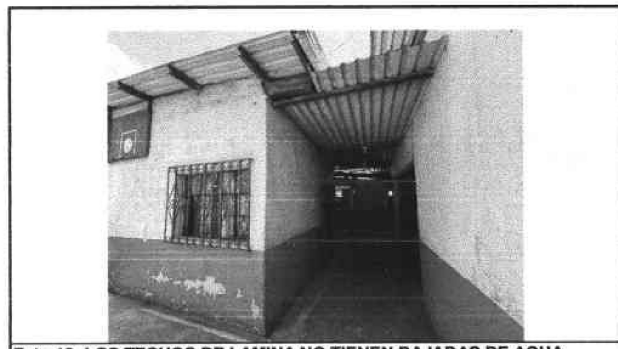
Foto 12: LOS TECHOS DE LAMINA NO TIENEN BAJADAS DE AGUA PLUVIAL NI CACAL, PINTURA EN MAL ESTADO, ESTRUCTURA METALICA CORROIDA
