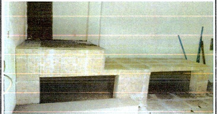
Foto 8: 20 REPARACION DE COCINA 20.2 SUSTITUCION DE ESTUFA RURAL (COMPLETA) INCLUYE CHIMENEA Y PLANCHA DE METAL
