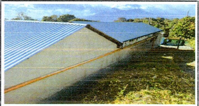
Foto 4: 7 CANALES Y BAJADAS DE AGUA PLUVIAL 7.3 REPARACION DE BAJADA DE AGUA PLUVIAL, TUBO PVC 3"
