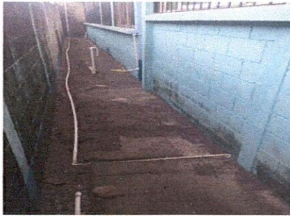
Foto 1: 14.9. Sustitución de tubería línea principal de red de agua potable.
