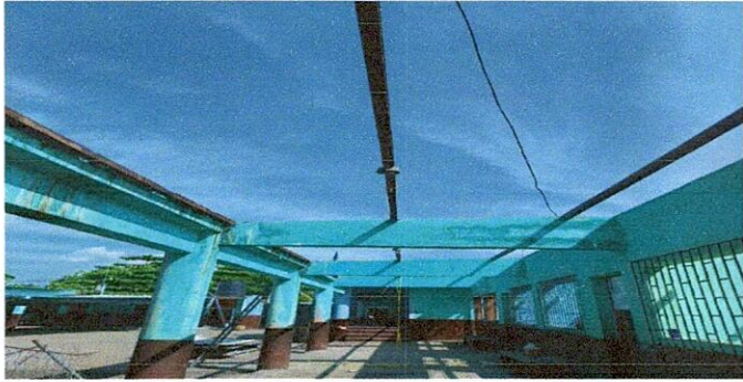
Foto1: DESINSTALACION DE LÁMINA EXISTENTE POR LÁMINA TROQUELADA ALUZINC 26
