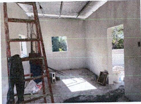
Foto 15: Reparación de repello y cernido en paredes
