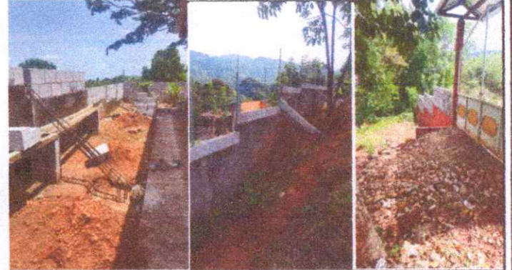
Foto 18, 19 y 20: reparación de muro perimetral de block y reparación de tubo hg malla galvanizada
