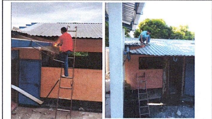
Foto 1: Sustitución de lámina, por lámina troquelada aluzinc calibre 26, Capote y de elementos de fijación.
