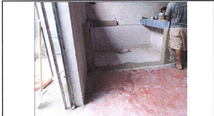
Foto 5: Sustitución de tubería PVC línea principal aguas negras, Sustitución de caja de registro, Sustitución de tubería línea principal, y Sustitución de chorro.
