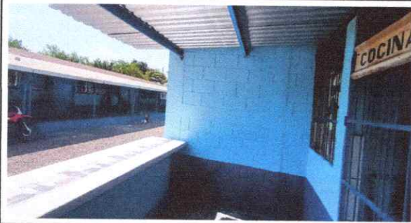
FOTO 1: Sustitución de lámina, por lámina troquelada aluzinc calibre 26. En el area de cocina.
