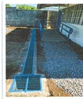
Foto 6: elaboracion de cunetas por filtracion de agua en los Modulos
