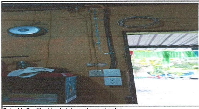
Foto 11: Sustitución de interruptores simples
