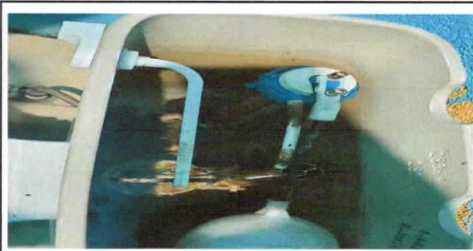
FOTO 10: SUSTITUCIÓN DE ACCESORIOS DE INODORO
