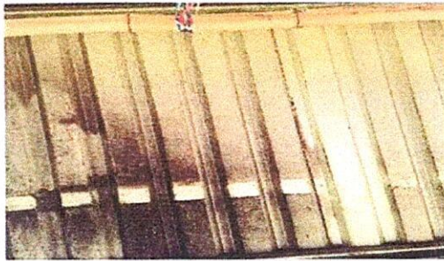
Foto1: sustitución de lámina troquelada aluzinc calibre 26
