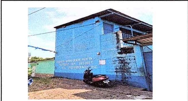
Foto1: Sustitución de lámina, por lámina troquelada aluzinc calibre 26° segundo nivel y pintura de exterior de escuela.
