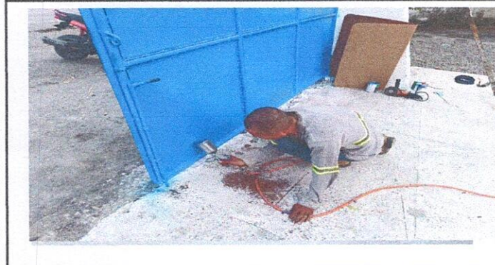
Foto 3: 12.1 Mantenimiento a portones de metal. Proceso durante la reparación del portón, despues de lijado, aplicación de pintura anticorrosiva
