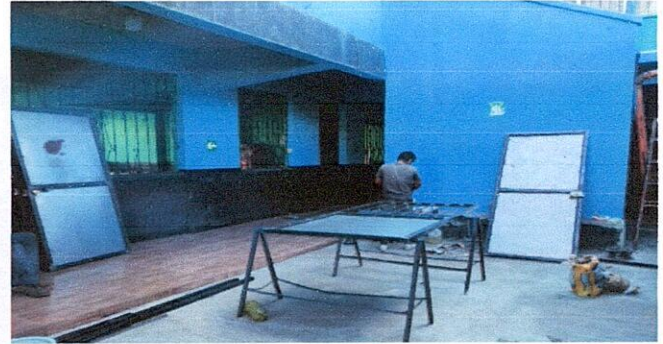
Foto 20: Sustitución de puerta, de las gradas del segundo nivel
