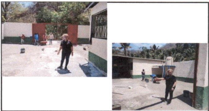
Foto 6: LOSA DE PATIO. SUSTITUCIÓN DE PISO DE TORTA DE CONCRETO.
