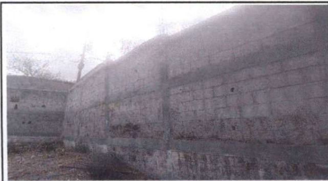
Foto 1: Muro perimetral de block en malas condiciones, peligro para estudiantes y maestros
