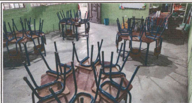
FOTO 1: AULA 2 REPARACIÓN DE PISO DE TORTA DE CONCRETO E INSTALACIÓN DE PISO CERÁMICO
