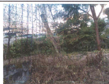
Foto 4: Muro colapsado, malla metalica detenida en árboles
