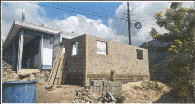
Foto1: Finalización del levantado de muro para el aula.
