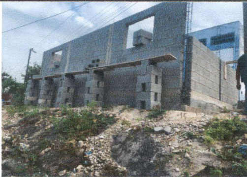
Foto 3: Levantado de muros del aula, hasta altura de techo.
