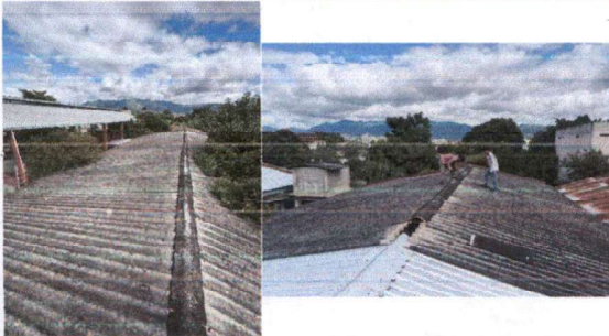
Foto1: Sustitución de duralita en mal estado en siete aulas del módulo uno y dos aulas del módulo dos del edificio escolar.
