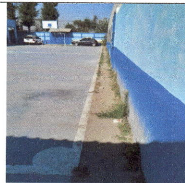
Foto 2 Colocación de red de drenaje aguas pluviales (Reparación de red de drenaje y red de agua potable)
