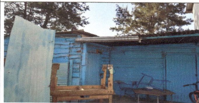
Foto 1 Sustitución de costaneras de 4 x 4 pulgadas para columnas (Estructura de techo)
