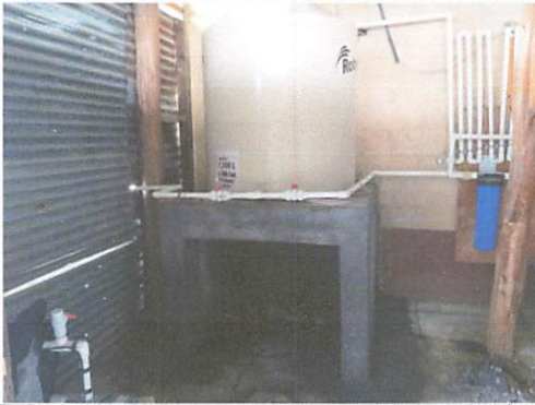
Foto 1: Base de tinaco finalizado, ahora si, mas resistente
