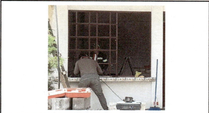
Renglón 5: colocación de azulejo en despachador de alimentos.
