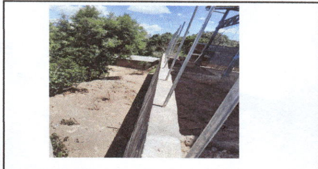
Foto 2: Finalización del muro de contención
