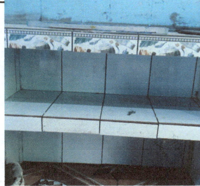
Foto 2: Construcción de Gabinete de concreto mas azulejo exterior de dos espacios 2.50 x 60 de fondo x 85 de alto.
