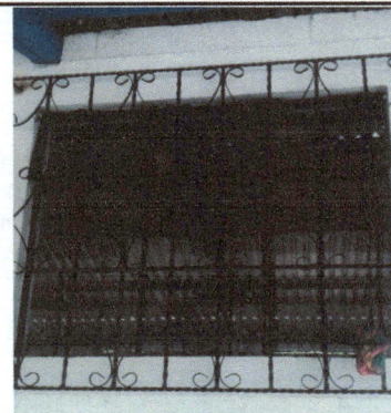
Foto 2: Trabajo y elaboración de balcones de 145x140 hierro entorchado y pintura.
