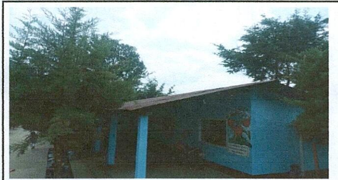
Foto1: Sustitución de Techo de cocina con lamina Troquelada Alucink calibre 26
