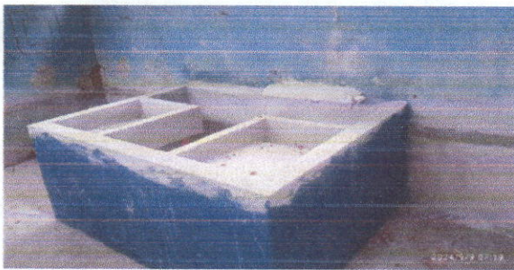
Foto 3: SUSTITUCION DE PILAS DETERIORADOS EXISTENTES, A PILA FABRICADO DE CONCRETO ARMADO CON REFUERZO ELECTROMALLA
