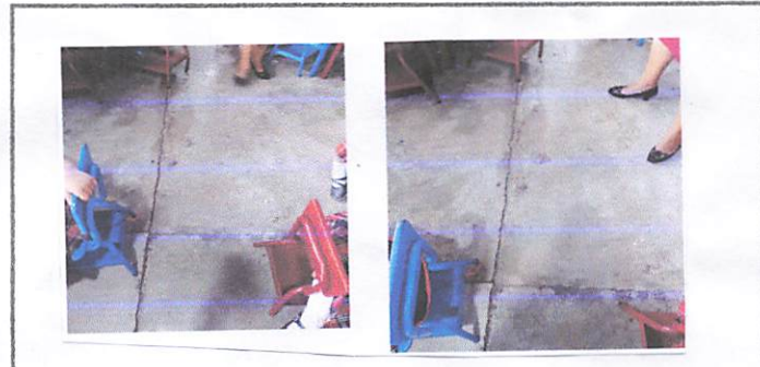
Foto 6: Piso: En el aula la torta se está agrietando y está undida en algunas partes se fundirá nuevamente y se colocará piso cerámico anti deslizante.
