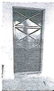
Foto 3. Fabricación e instalación de puerta de metal de 2.30x1 en salón de computación.
