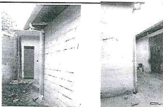
Foto 5: Sustitución de bajada de agua pluvial de metal por tubo PVC de 3"
