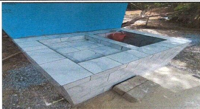
Foto7: Instalación de azulejos en la pila (Renglón de trabajo No. 6.1.)
