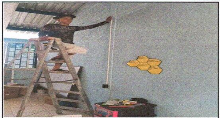
Foto 14: Sustitución de ducto electrico mas accesorios (Renglón de trabajo 8.4.)
