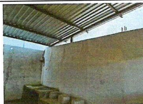
Foto 12: Reparacion de Muro en cocina (sellado de agujero en pared y levantado de hiladas de block)
