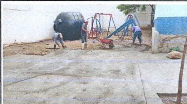
Foto 4: Sustitución de piso de torta de concreto en área de juegos
