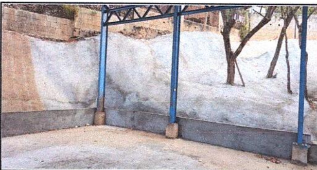
Foto 5: Levantamiento de 3 hiladas de block con repello y cernido para evitar que el agua ingrese en el área afectada y se haga charco con lodo, ya que es la entrada principal al establecimiento educativo.
