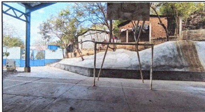
foto2.proteccion de muro, elaboracion de 3 hiladas de block,instalacion de cuneta de concreto para proteccion del establecimiento educativo.
