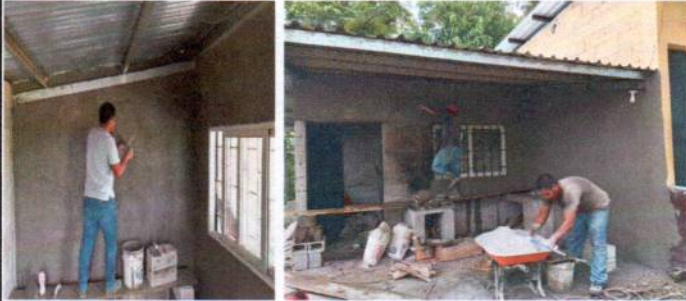
Foto1: Aplicación de repello en paredes de cocina exterior e interior
