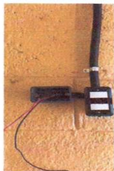
Foto 17: Instalación de apagador doble
